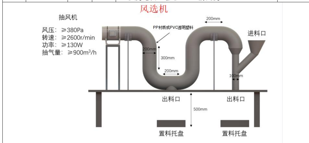
图 1 风选机设计示意图
